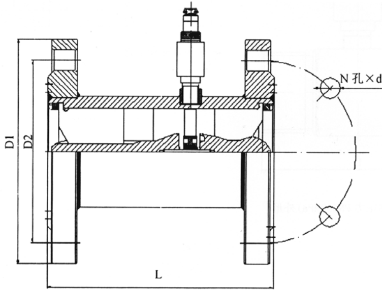
图4 DN40~300外形
